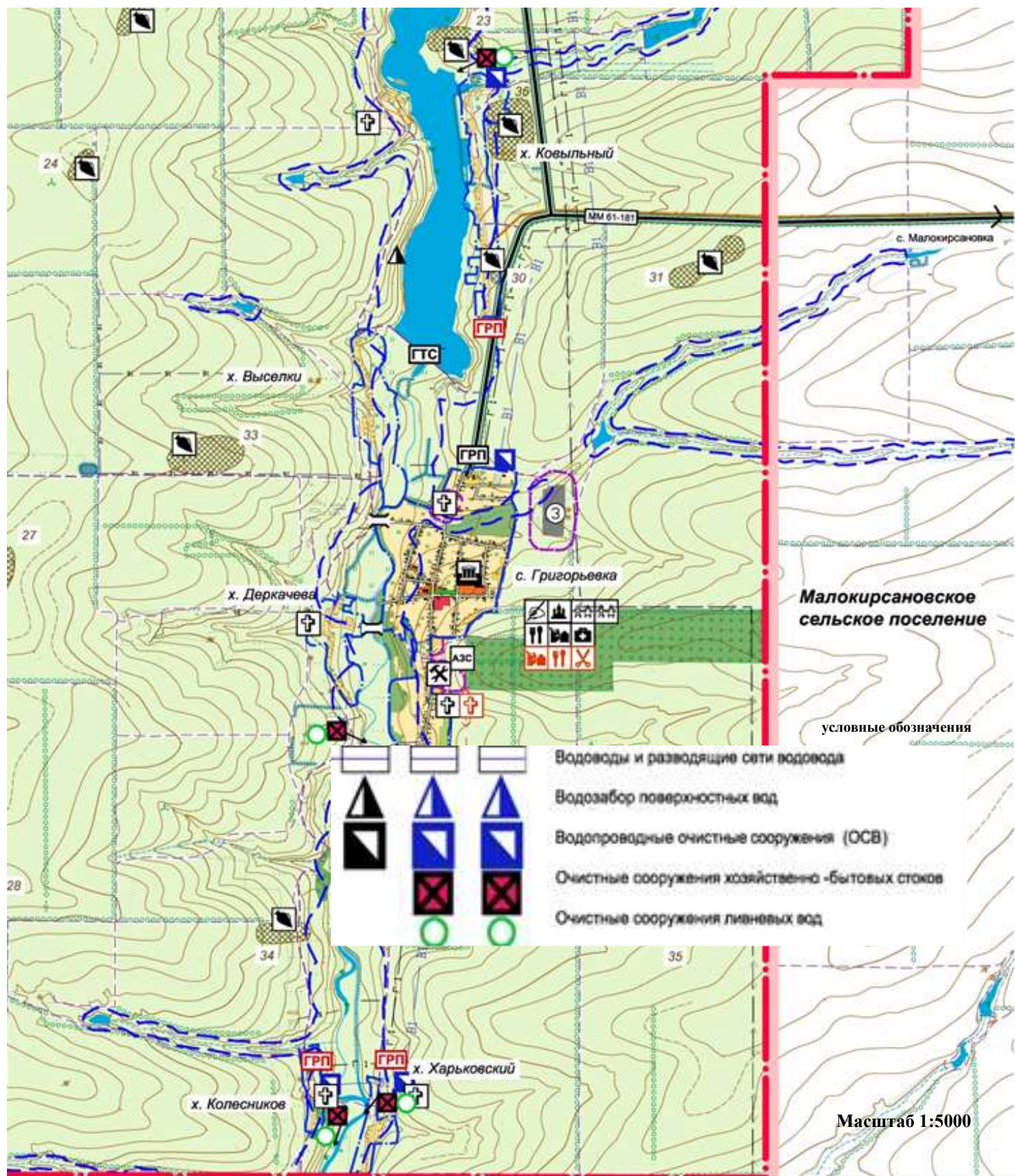
Приложение 23 Перспективная схема водоснабжения и водоотведения х. Ковыльный, х. Выселки, с. Григорьевка, х. Деркачева, х. Харьковский, х. Колесников
